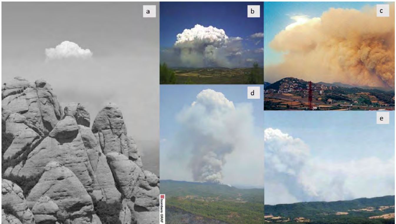
Pirocúmul·s d'incendis extrems a Catalunya. a) Castelltallat, 1994, des de Montserrat. b) Cardona, 2005. c) Berguedà, 1994. d) Sant Llorenç Savall, l'11 d'agost del 2003. e) Solsonès, 1998, que va cremar 22.000 ha el 19 de juliol fins ben entrada la nit del 20 de juliol.
